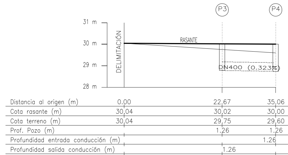
Perfil Longitudinal 2 - C./Pintor Benedito Sur
