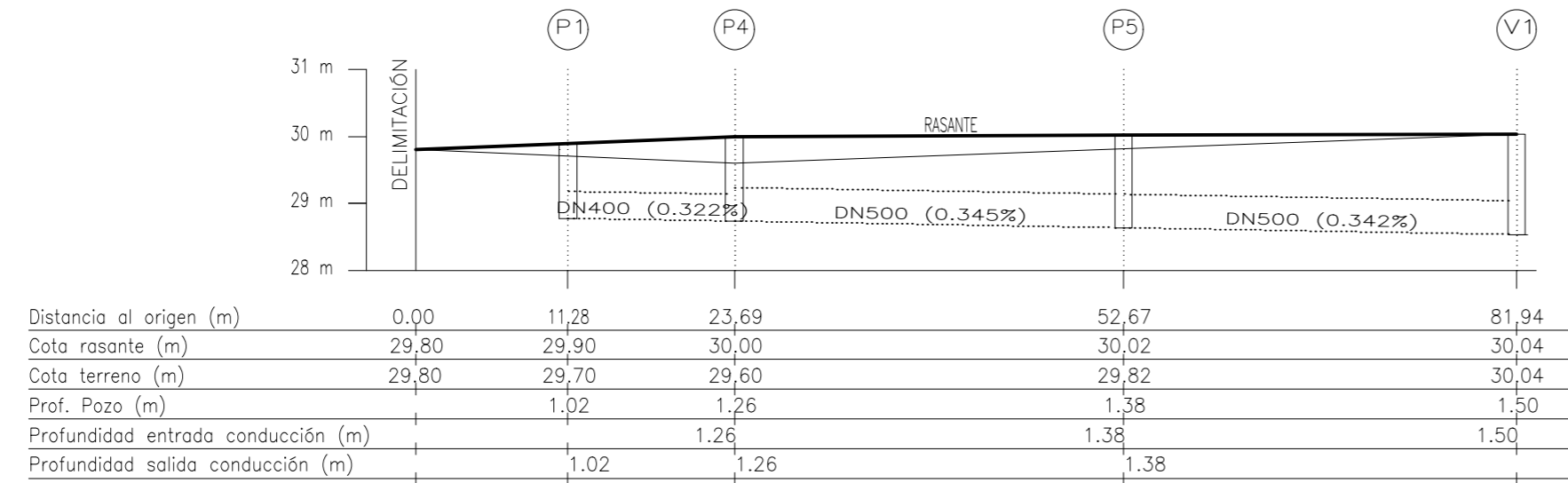
Perfil Longitudinal 1 - C./Poeta Llorente
